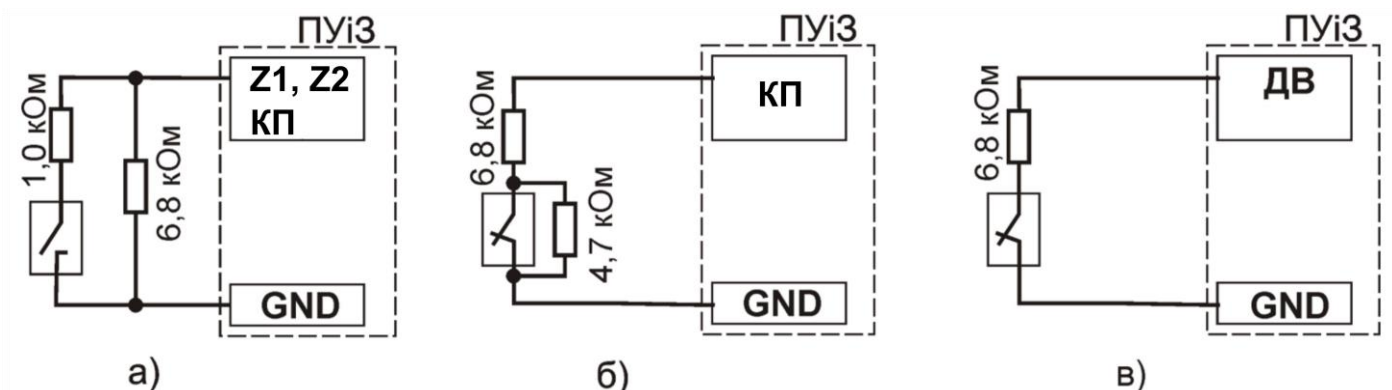
Рисунок А.1 – Підключення входів та виходів
