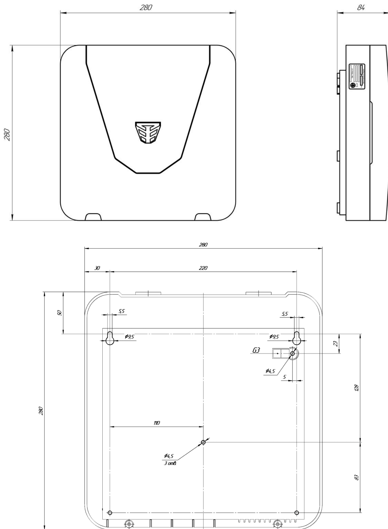
Рисунок Б.1 – Установчі розміри ППКО
