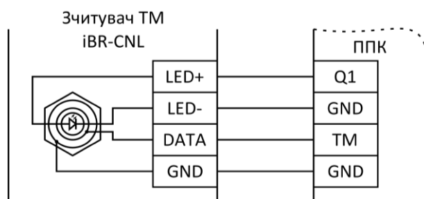
Рисунок 2.11 – Схема підключення зчитувача ключів ТМ
