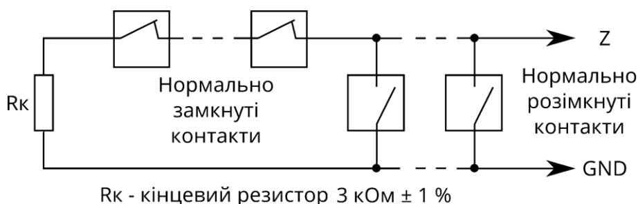
Рисунок 2.7 – Схема підключення охоронних датчиків з нормально замкнутими та нормально розімкнутими контактами
