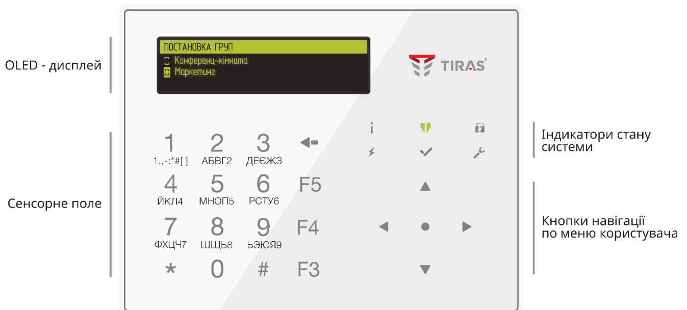
Рисунок 5.3 – Клавіатура K-GLCD
