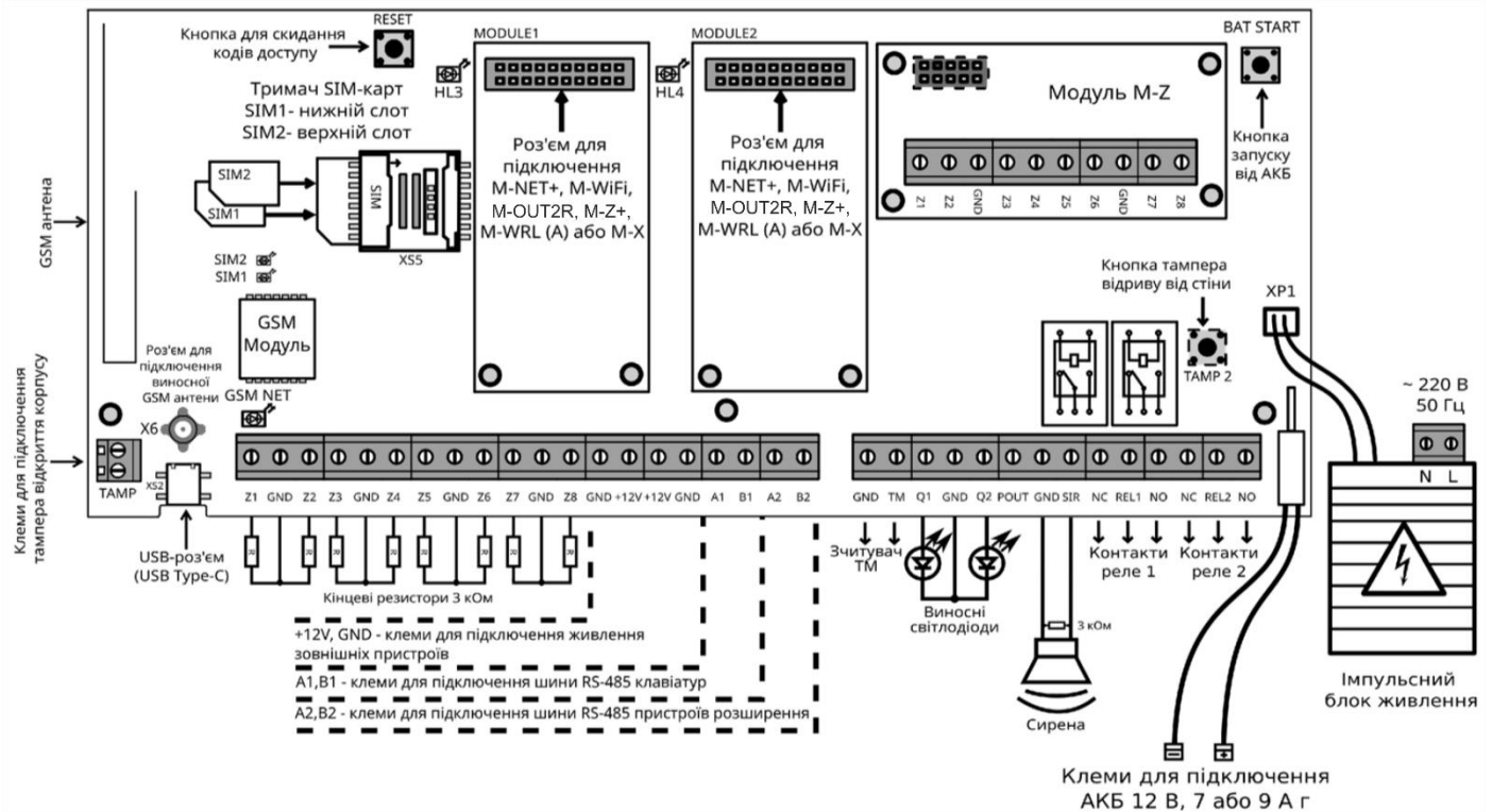
Рисунок А.1 – Схема електрична підключення ППКО Orion NOVA L HW3
