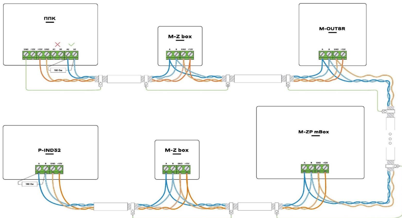
Рисунок 2.5 – Приклад підключення виносних модулів (варіант ППКО на початку лінії обміну)
