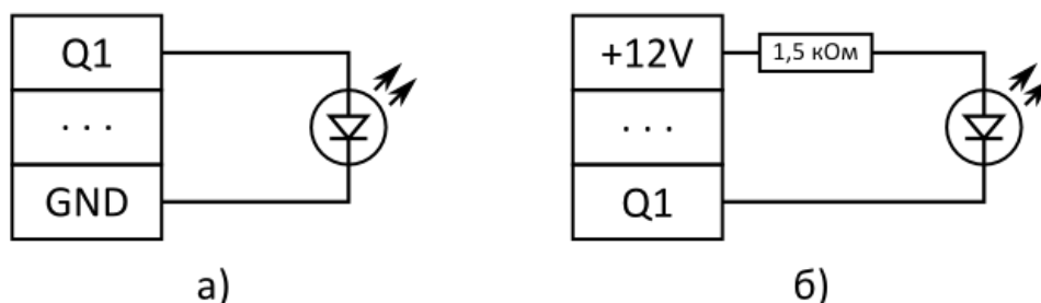
Рисунок 2.10 – Схеми підключення індикаторів підтвердження
