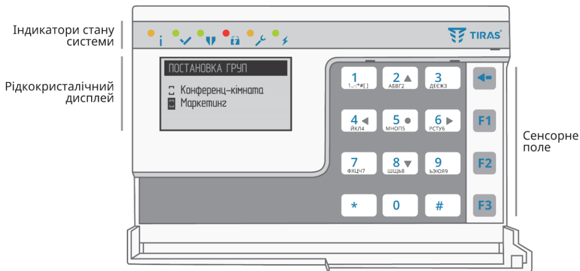
Рисунок 5.1 – Клавіатура K-LCD
