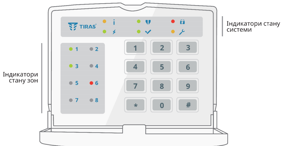
Рисунок 5.4 – Клавіатура K-LED8
