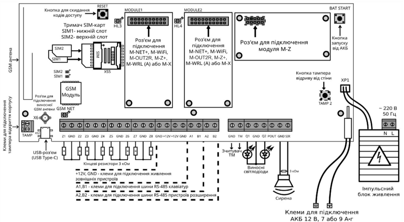
Рисунок А.2 – Схема електрична підключення ППКО Orion NOVA M HW3
