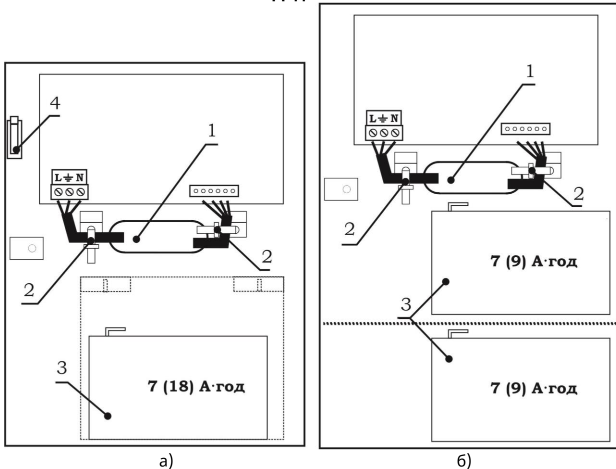
Рисунок В.1 – Компоновка БЖ1230 (а) та БЖ2415 (б):
