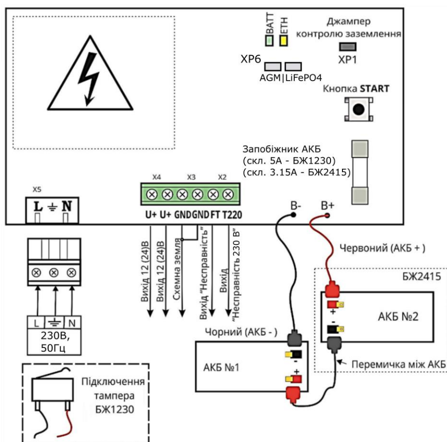
Рисунок А.2 – Підключення входів та виходів
