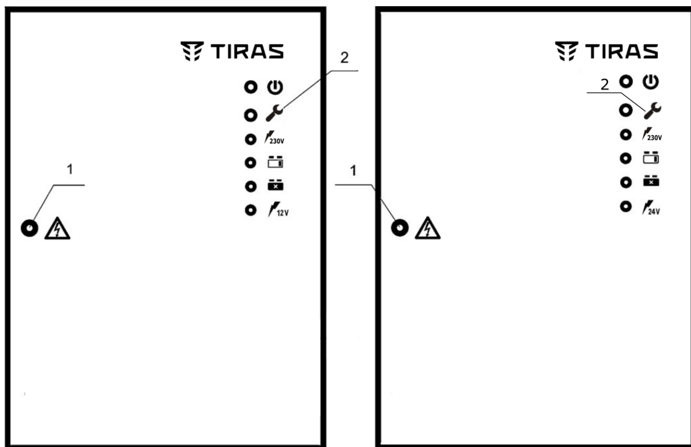
Рисунок А.1 – Зовнішній вигляд БЖ1230 (а) та БЖ2415 (б): 1 – гвинт фіксації дверей; 2 – індикатори режимів роботи.
