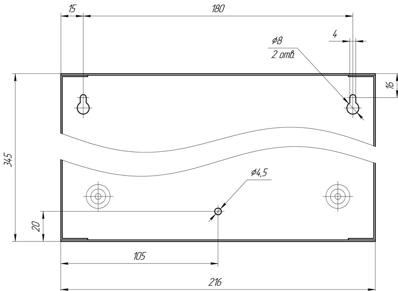
Рисунок Б.2 – Розмітка отворів для кріплення БЖ2415
