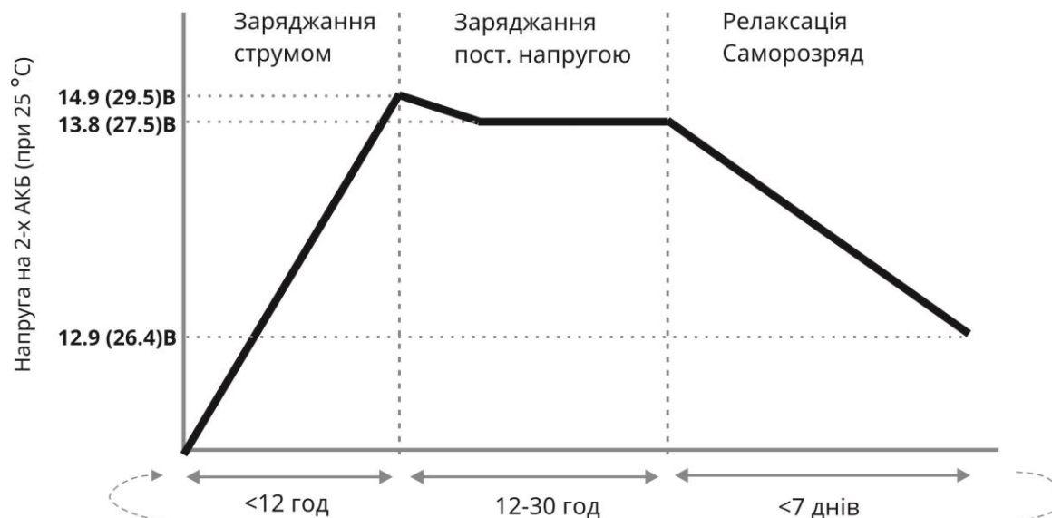
Рисунок 3.1 – Цикли роботи зарядного пристрою
