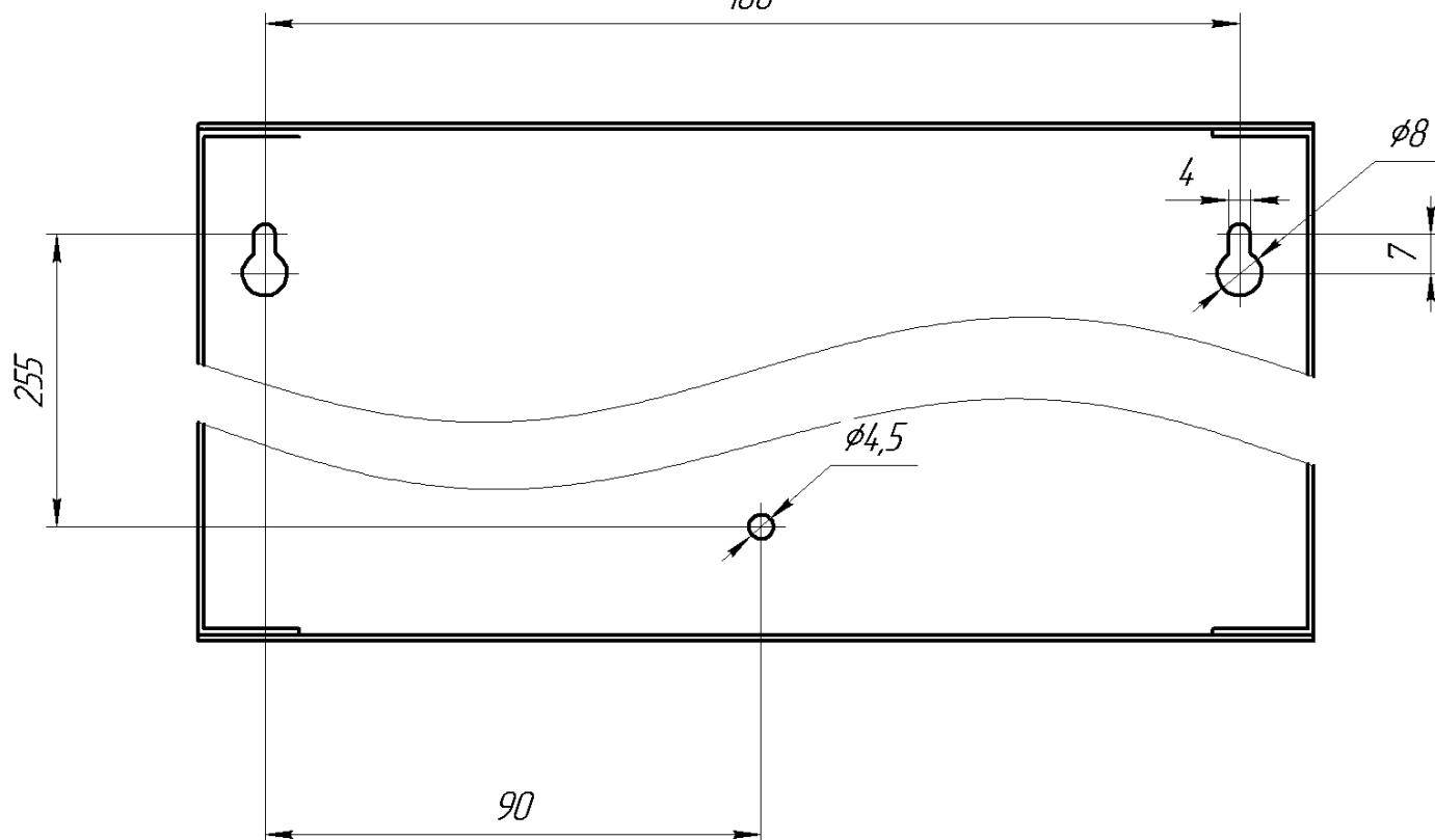
Рисунок Б.1 – Розмітка отворів для кріплення БЖ1230
