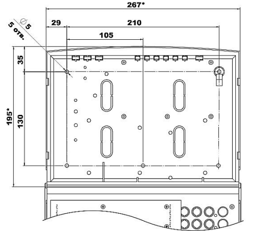
Рисунок 4.1 – Розмітка отворів для кріплення панелі
