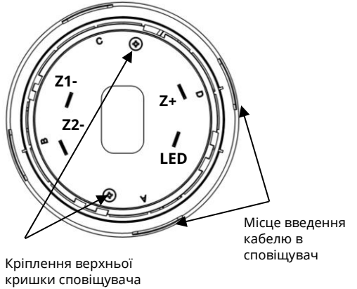
Рисунок 4.1 – Вигляд сповіщувача з боку контактів
