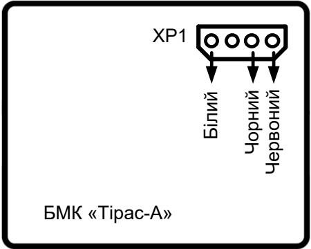
Рисунок 2.5 – Підключення БЖ до БМК «Тірас-А»
