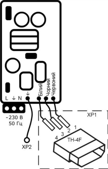
Рисунок 2.1 – Зовнішній вигляд БЖ
