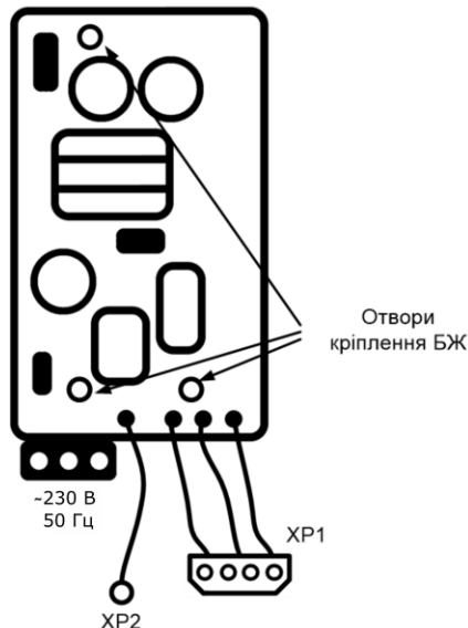
Рисунок 2.6 – Отвори кріплення БЖ
