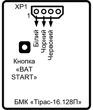
Рисунок 2.3 – Підключення БЖ до БМК «Тірас-16.128П» із кнопкою «BAT START»
