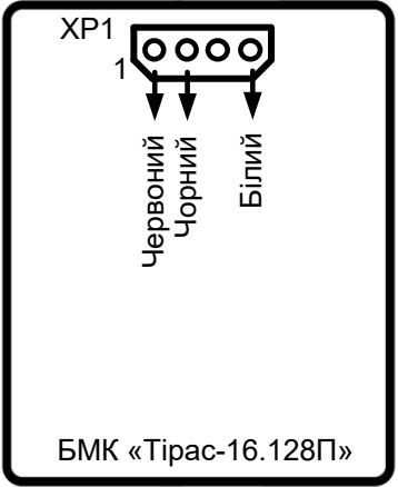
Рисунок 2.4 – Підключення БЖ до БМК «Тірас-16.128П» без кнопки «BAT START»
