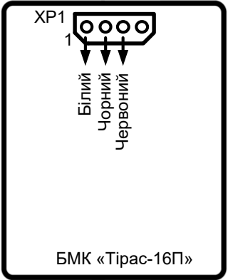
Рисунок 2.2 – Підключення БЖ до БМК «Тірас-16П»
