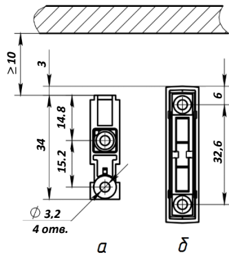
Рисунок 3.3 – Установчі розміри для датчика та магніту
