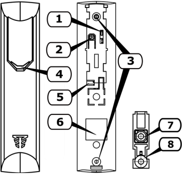
Рисунок 3.4 - Зовнішній вигляд елементів датчика 1 – Кнопка тампера, 2 – Кнопка «Старт», 3 – Гвинти корпусу, 4 – Світлодіодний індикатор, 5 – Отвір для дротів виносного геркона, 6 – QR-код для приписування, 7 – Відривний елемент, 8 – Кронштейн Серійний номер використовується для приписування датчика до ППКО за допомогою програмного забезпечення (далі – ПЗ) oLoader II або застосунку Control NOVA II.
