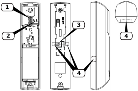
Рисунок 3.1 – Розміщення клемного з’єднувача, місць для прокладання дротів та вирізів 1 – Антена, 2 – Клемний з’єднувач, 3 – Місця для прокладання дроту, 4 – Місця для вирізів
