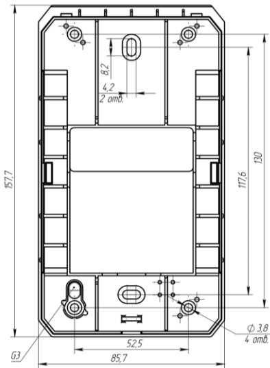
Рисунок 3.1 – Установчі розміри клавіатури
