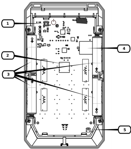
Рисунок 3.2 - Опис елементів клавіатури 1 – кнопка «Старт»; 2 – QR-код для приписування; 3 – елементи живлення; 4 – зумер; 5 – кнопка тампера
