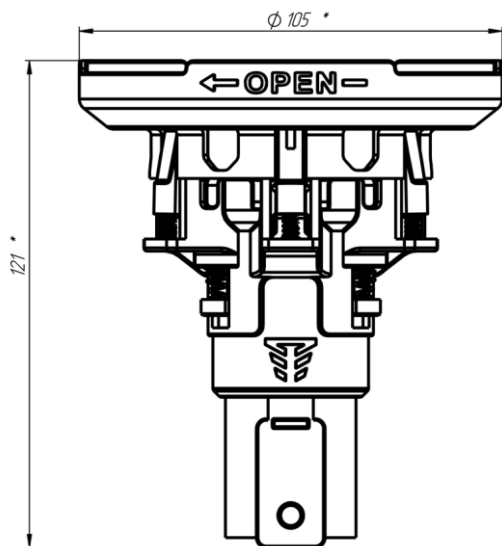
Рисунок 1.1 – Габаритні розміри знімача
