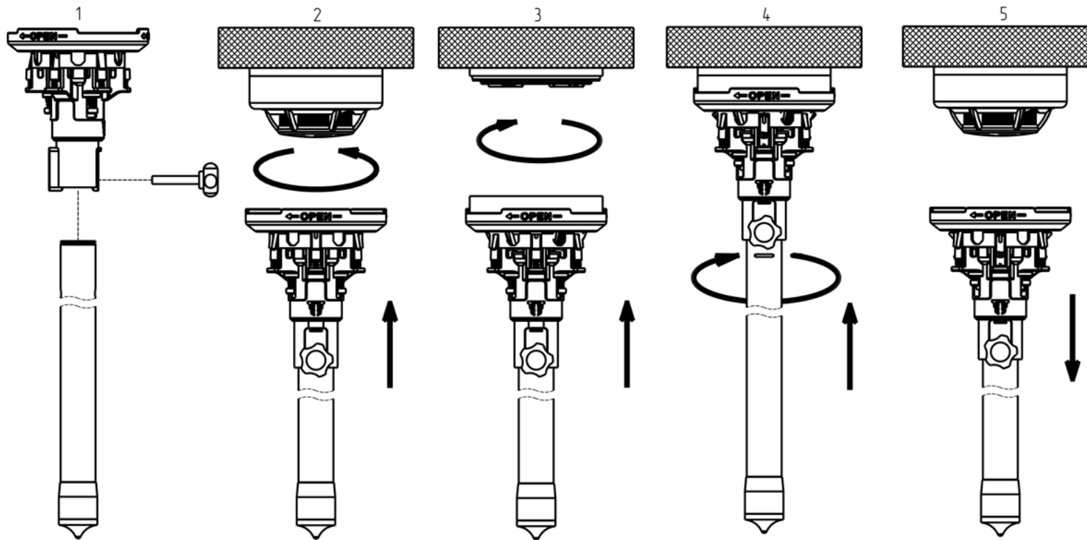
Рисунок А.1 – Зовнішній вигляд елементів знімача
