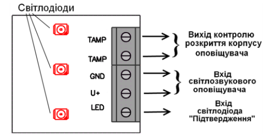
Рисунок 2.2 – Схема підключення оповіщувача
