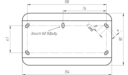
Рисунок 2.1 – Розмітка отворів на основі корпуса оповіщувача
