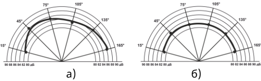
Рисунок 1.1 – Акустичні діаграми ОСЗ Джміль-1 (12/24V): а) – робоче положення, б) – повернене на 90° за годинниковою стрілкою положення
