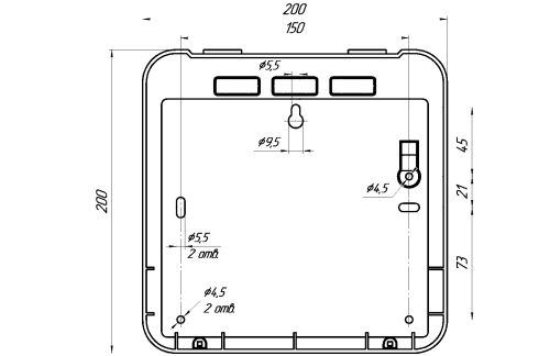
Рисунок 3.1 – Розмітка отворів для кріплення корпусу модуля
