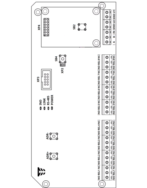
Рисунок 3.2 – Зовнішній вигляд плати модуля
