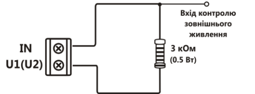
Рисунок 3.3 – Схема підключення входу IN
