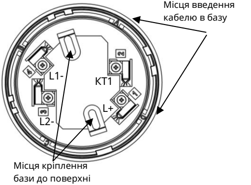
Рисунок 4.1 – Розташування клем на базі СПКА
