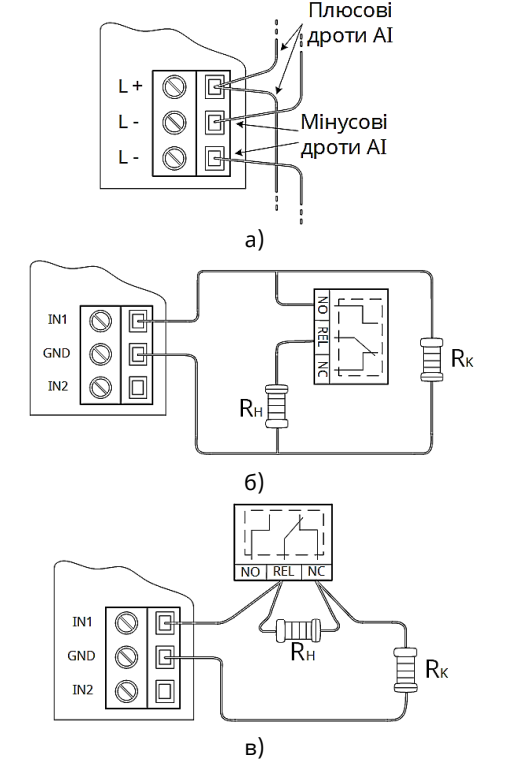
Рисунок 4.1 – Схеми підключень зовнішніх кіл до входів пристрою
