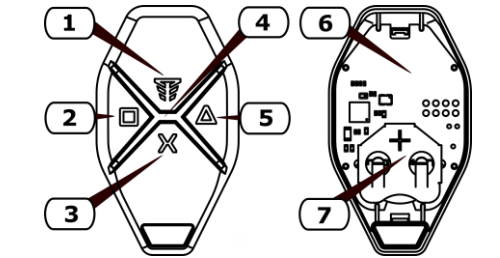
Рисунок 3.1 – Зовнішній вигляд елементів брелока 1 - постановка під охорону; 2 - постановка в режимі «Я вдома»; 3 - зняття з охорони; 4 - світлодіодний індикатор; 5 - «Тривожна кнопка» 1 ; 6 - плата брелока 7 - тримач елемента живлення.
