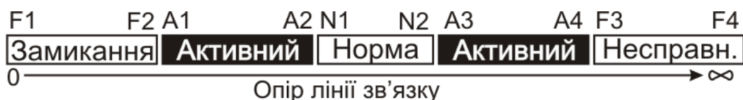
Рисунок 4.3 – Зміна стану контрольованих кіл зі зміною опору підключених ліній зв'язку
