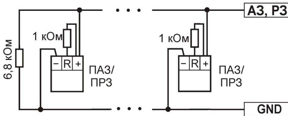
Рисунок А.3 – Підключення ПАЗ та ПРЗ до входів «А3» та «Р3» за двопровідною схемою (додаткові відомості з підключення – див. паспорт на ПАЗ або ПРЗ)
