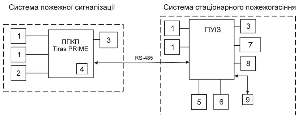
а) підключення ППКП ПУіЗ до ППКП «Tiras PRIME» та «Tiras PRIME A mini»
