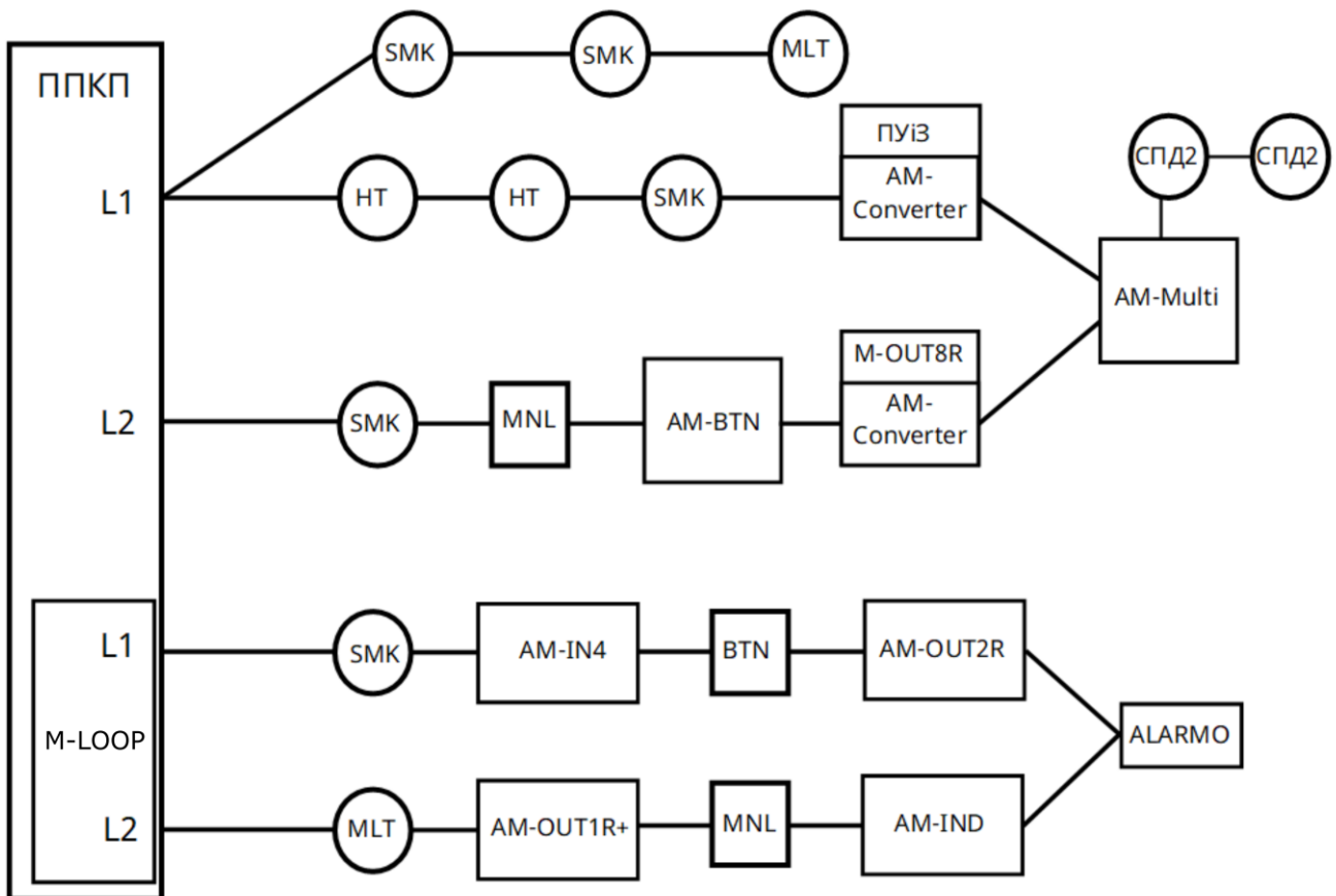
Рисунок 4.2.1 – Схема приєднання адресних компонентів до АІ
