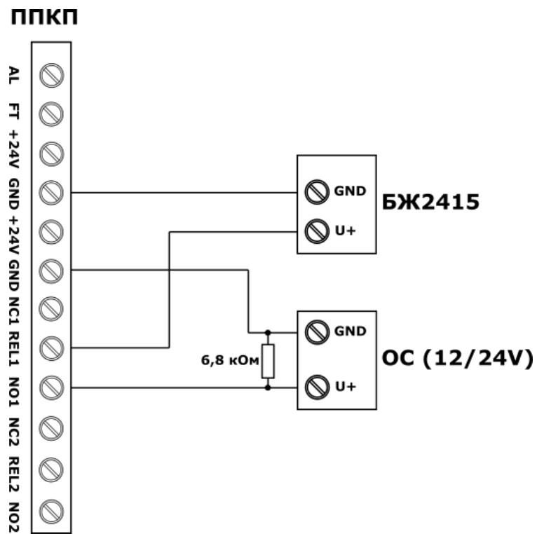
Рисунок Б.4 – Приклад підключення пристроїв оповіщення до виходів REL1, REL2
