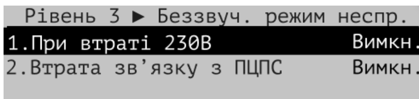
Рисунок 10.13.2 – Вікно налаштувань беззвучного режиму несправностей
