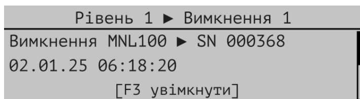
Рисунок 8.5.1 – Приклад вікна повідомлення режиму вимкнення
