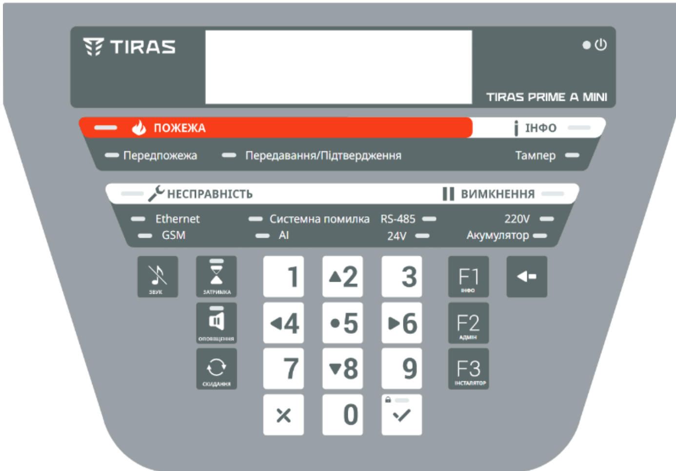
Рисунок 7.4 – Розташування кнопок та індикаторів на передній панелі ППКП
