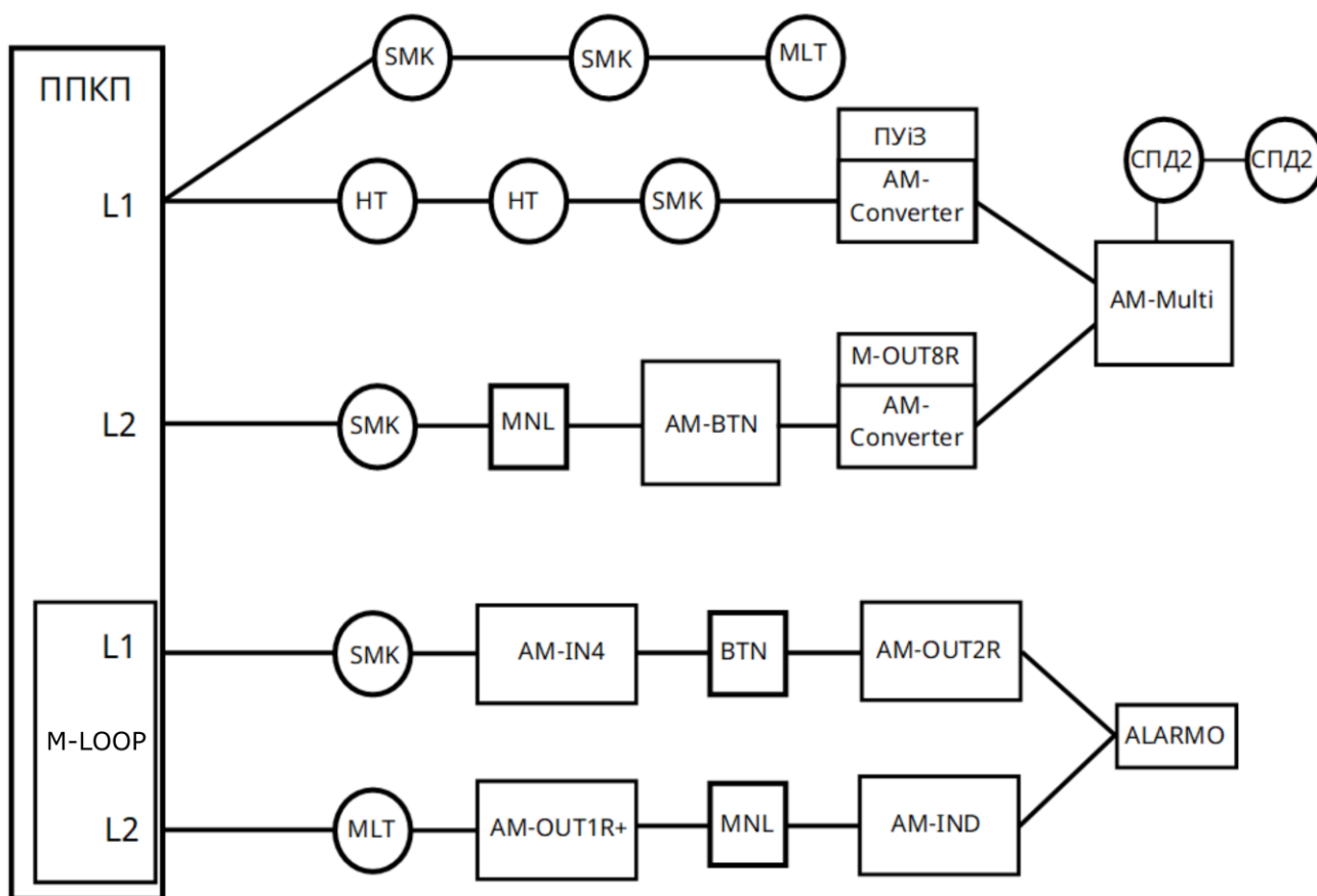
Рисунок 4.2.1 – Схема приєднання адресних компонентів до АІ
