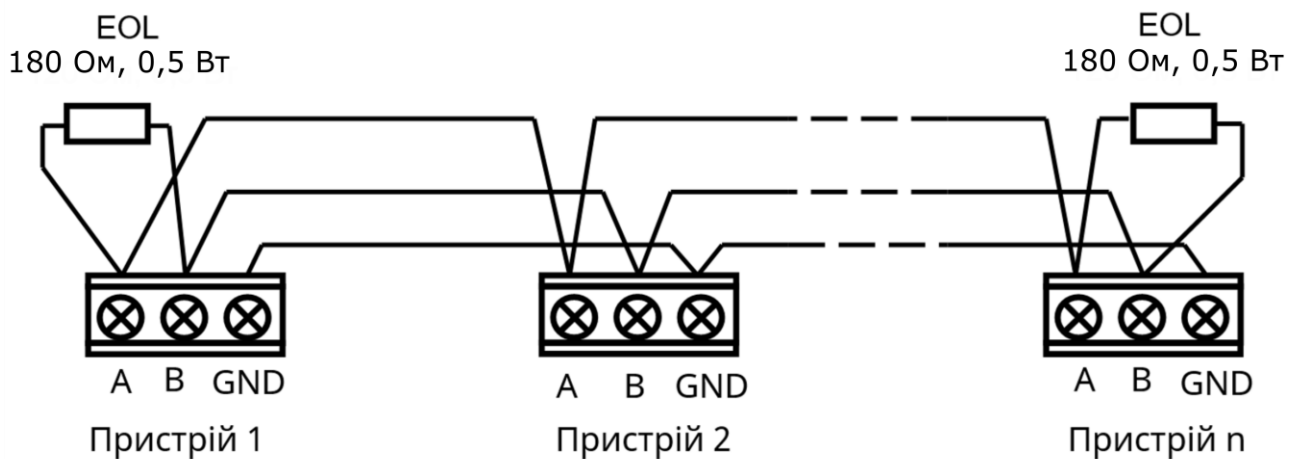
Рисунок 11.1.3 – Підключення до шини RS-485
