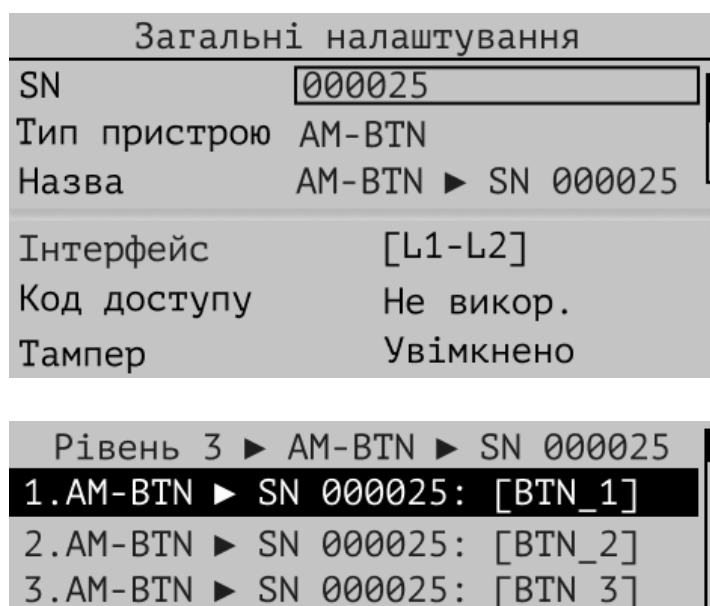
Рисунок 10.2.9 – Вікно для налаштування кнопок панелі AM-BTN
