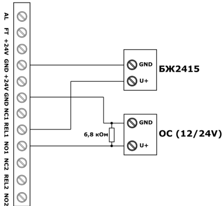
Рисунок Б.4 – Приклад підключення пристроїв оповіщення до виходів REL1, REL2
