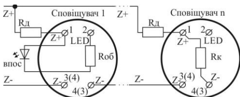
Рисунок 4.3 – Підключення ВПОС або світлодіода
