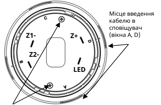
Кріплення верхньої кришки сповіщувача
