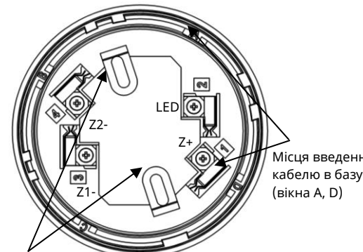
Місця введення кабелю в базу (вікна А, D)
