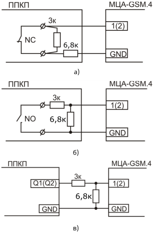
Рисунок 4.2 – Підключення параметричних входів «1» та «2»: а) до нормально замкнених виходів; б) до нормально розімкнених виходів; в) до виходів типу «відкритий колектор».
