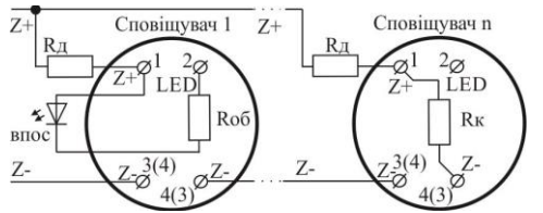
Рисунок 4.3 – Підключення ВПОС або світлодіода
