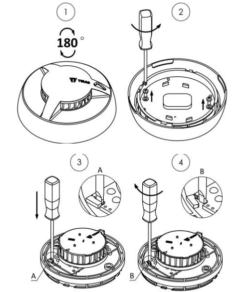
Рисунок 4.2 – Послідовність кроків для видалення ламкого елемента
