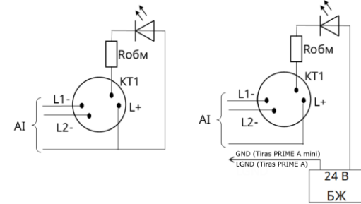
а) б) Рисунок 4.2 – Підключення ВПОС або світлодіода
