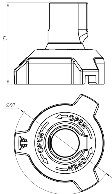
Рисунок 1.1 – Габаритні розміри знімача
