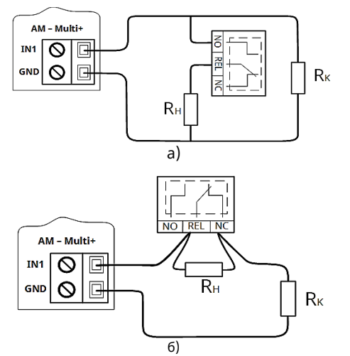
Рисунок 4.2 – Підключення входів IN: а) Схема підключення реле з NO контактом паралельно з кінцевим резистором R к . б) Схема підключення реле з NC контактом послідовно з кінцевим резистором R к .
