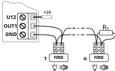
Рисунок 4.3 – Схема підключення виходів оповіщення
