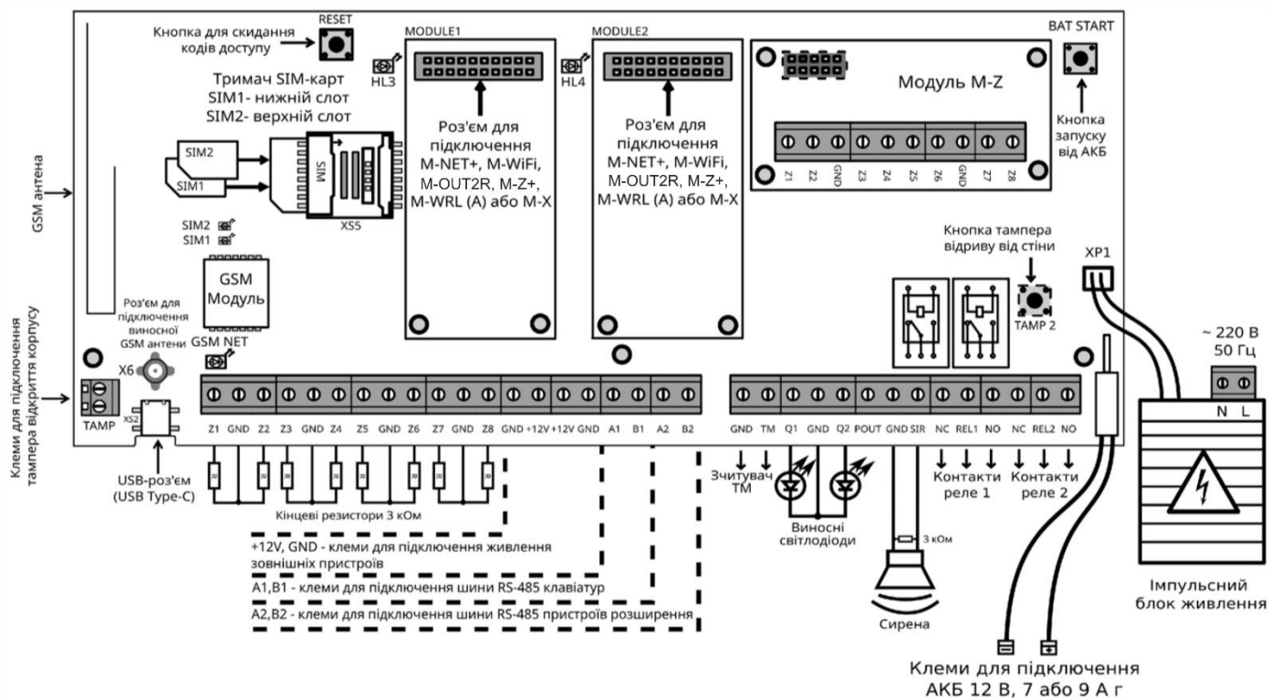
Рисунок А.1 – Схема електрична підключення ППК Orion NOVA L HW3
