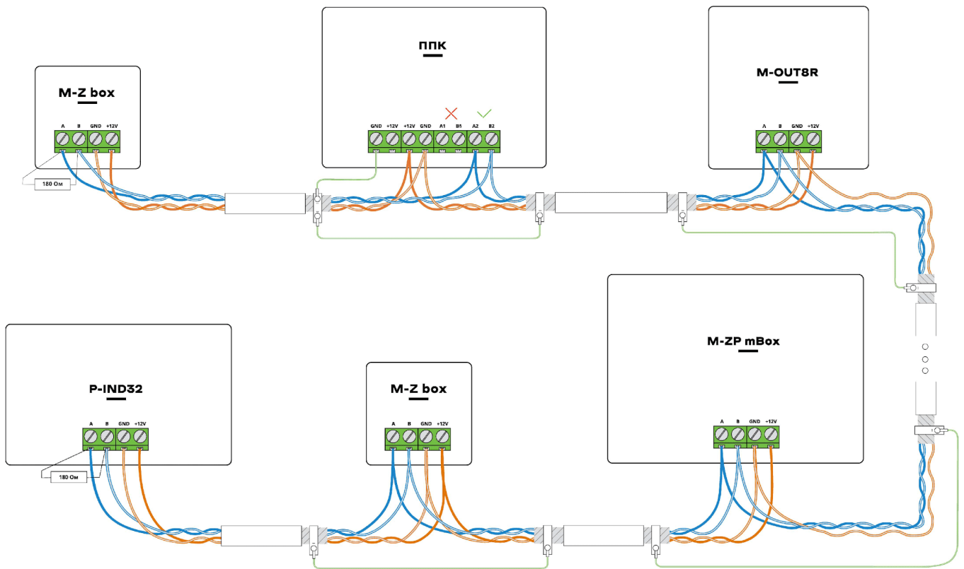
Рисунок 2.6 – Приклад підключення виносних модулів (варіант ППК всередині лінії обміну)
