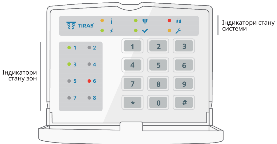
Рисунок 5.4 – Клавіатура K-LED8
