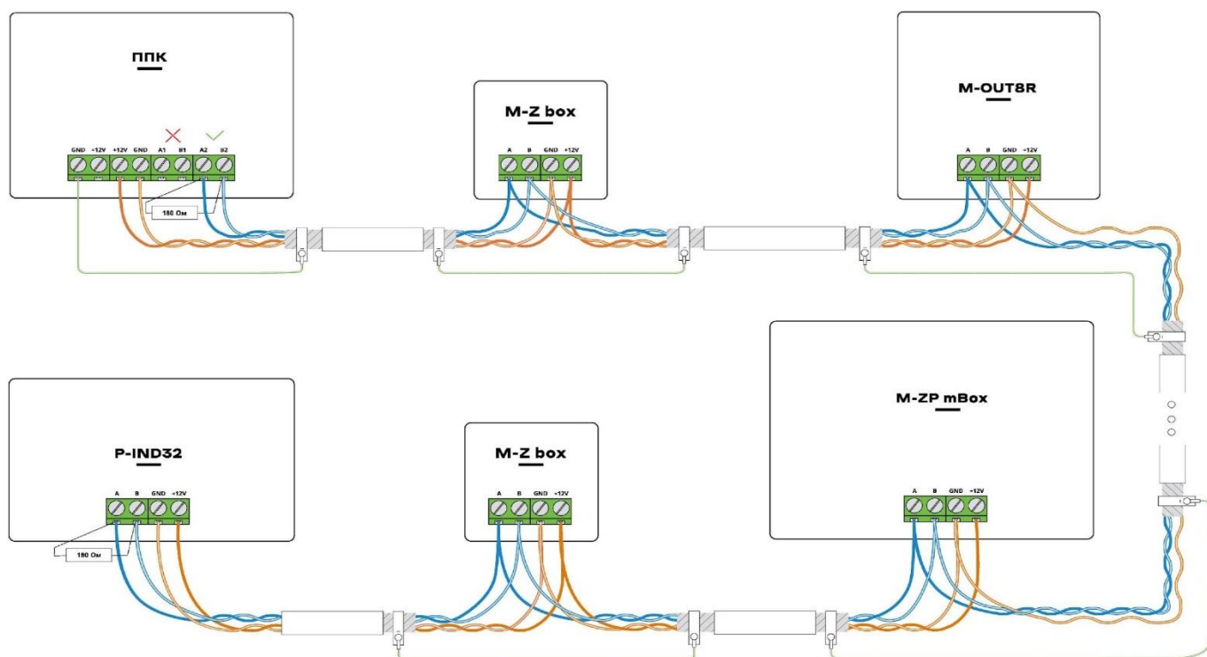
Рисунок 2.5 – Приклад підключення виносних модулів (варіант ППК на початку лінії обміну)
