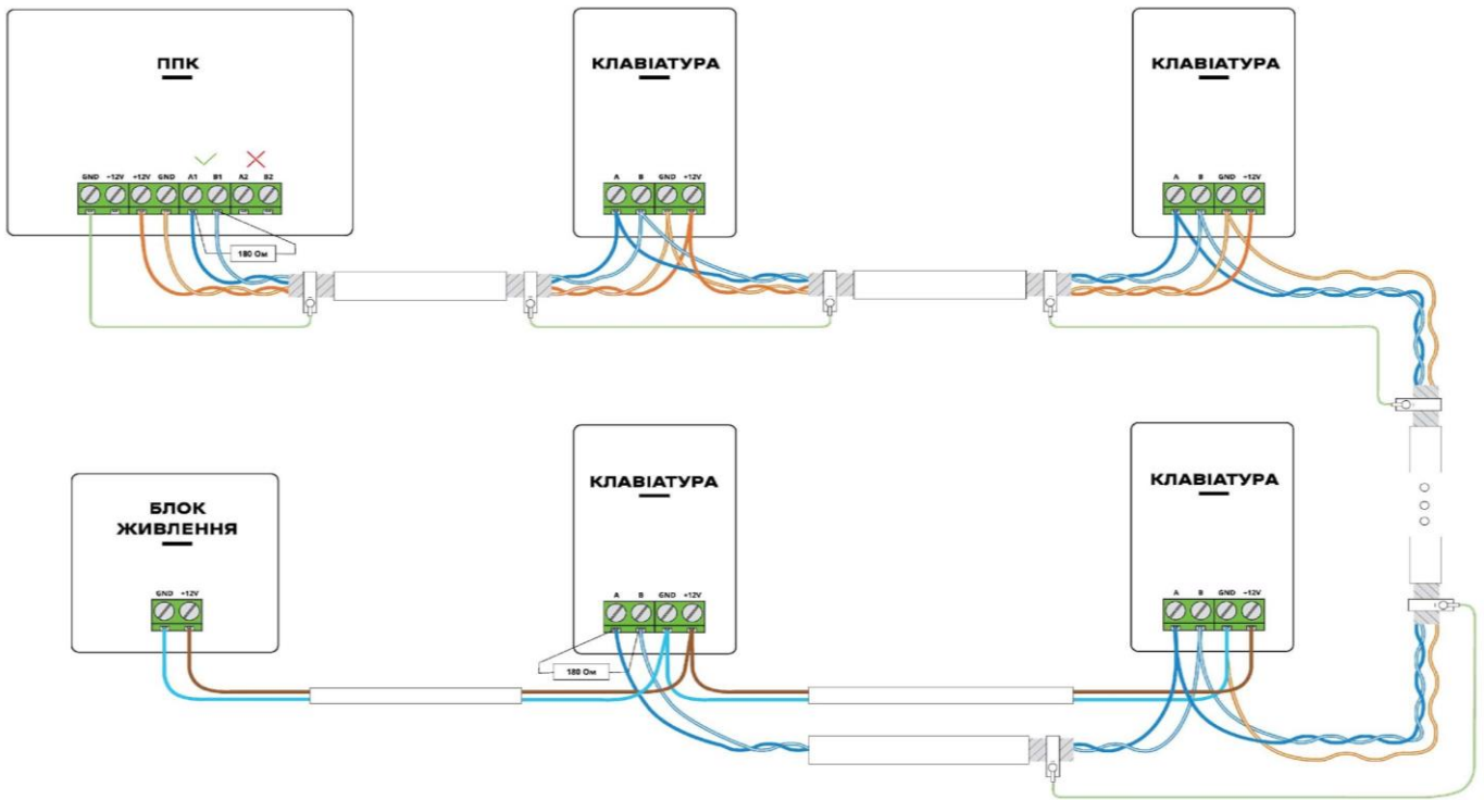
Рисунок 2.3 – Приклад підключення клавіатур (варіант ППК на початку лінії обміну)
