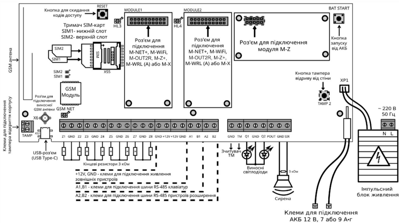
Рисунок А.2 – Схема електрична підключення ППК Orion NOVA M HW3
