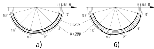
Рисунок 2 – Акустичні діаграми оповішувачів ОСЗ (24V):
