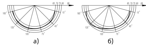
Рисунок 3 – Акустичні діаграми оповішувачів ОСЗ-Ех:
