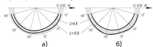
Рисунок 1 – Акустичні діаграми оповішувачів ОСЗ: а) – робоче положення, б) – повернене на 90 ° за годинниковою стрілкою положення
