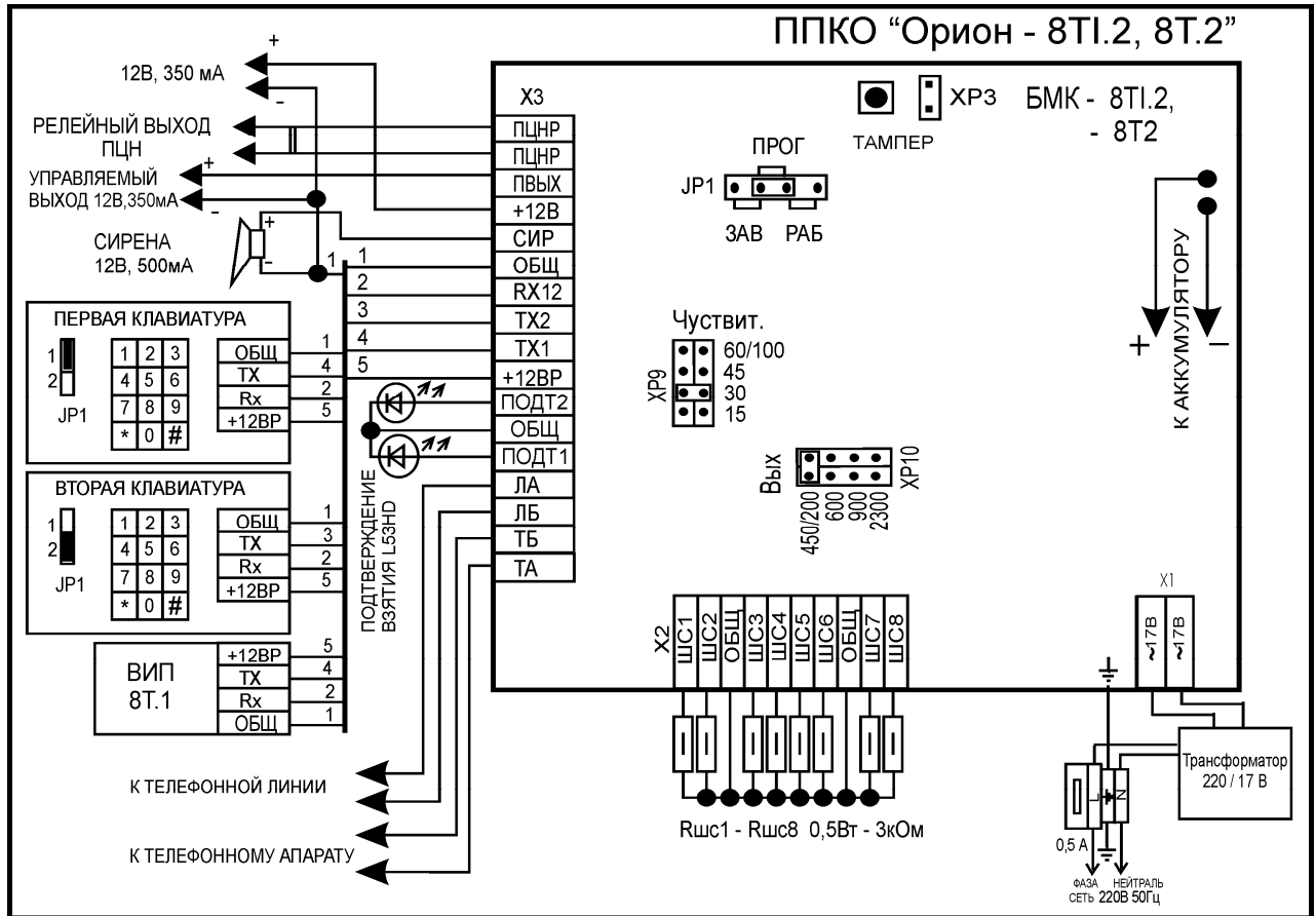
Малюнок А.1 Схема електрична підключення ХР3 встановлено в положенні, що блокує кнопку тампера
